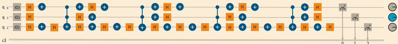
Aus dieser Quantenschaltung generiert das Composer-Panel direkt den dazugehörigen OpenQASM-Code für den Grover-Algorithmus (Abb. 8).
